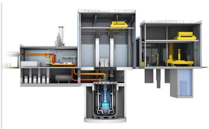
Sodium™ Reactor
